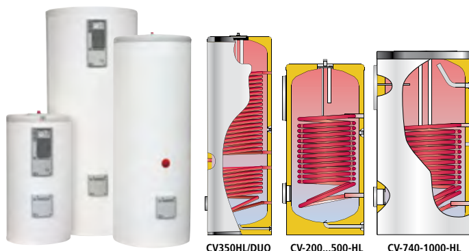
CV350HL/DUO
