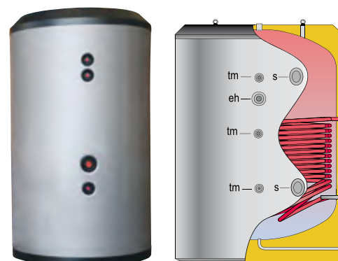
MV-1500-...5000-I-IB
